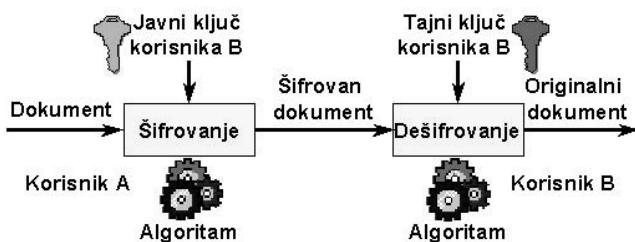
Slika 1: Asimetrična kriptografija 5
